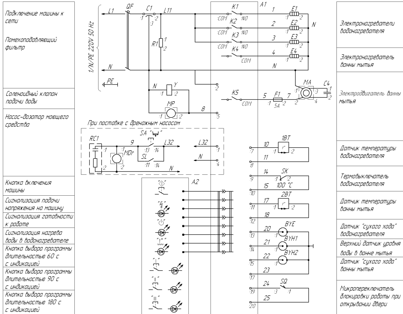
Схема машины МПФ-12-01-3
