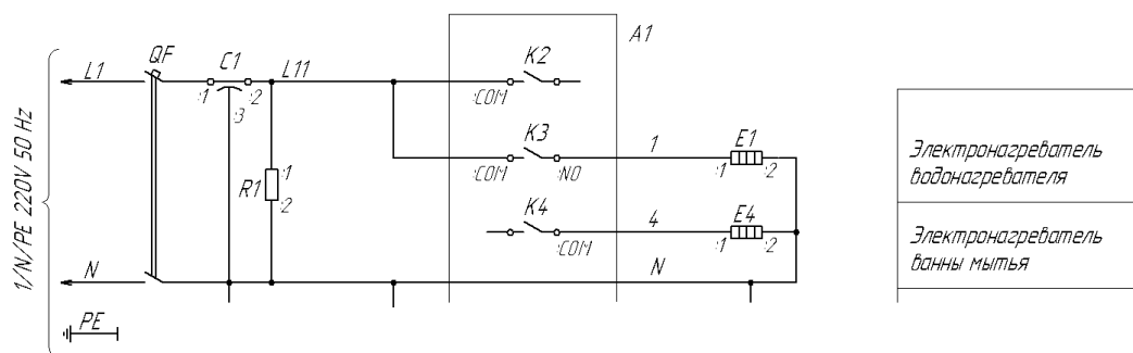
Рисунок 3 – Схема электрическая принципиальная
